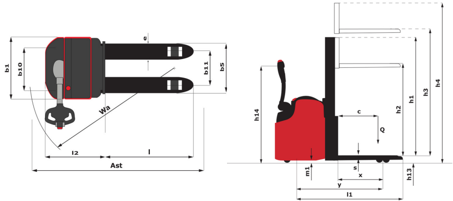
ES 412 ET - Dimensional drawing
