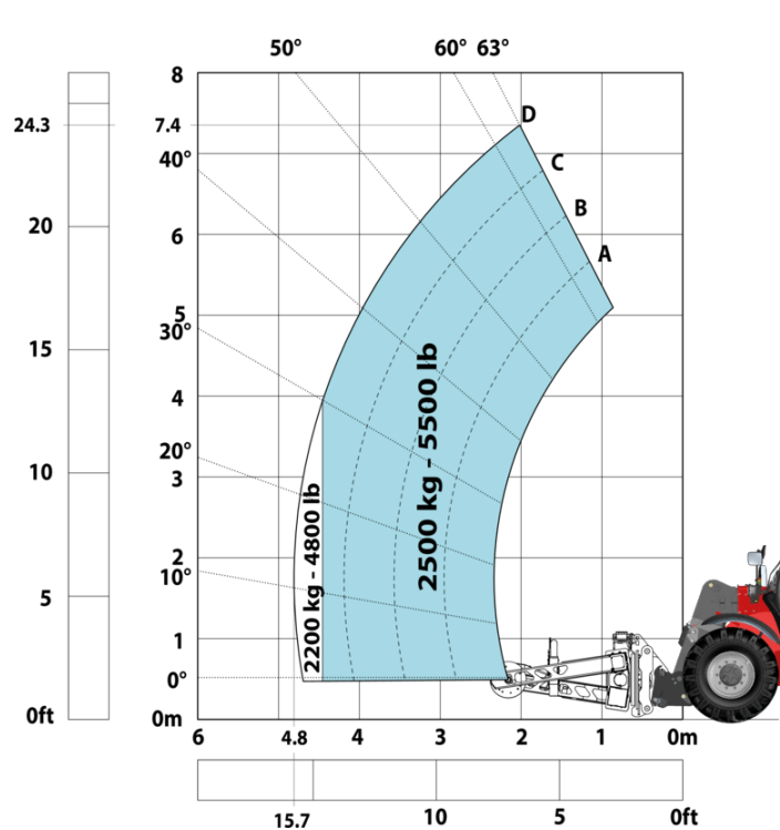
Machine op banden met bandenafnemer TH 49 (Metrisch)
