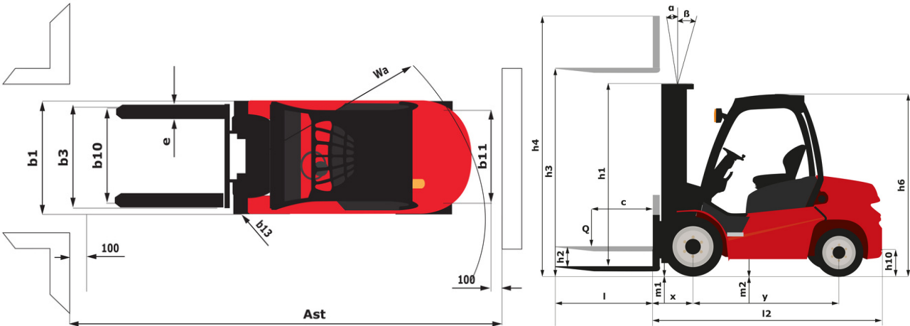
MI-X 35 G - габаритный чертеж
