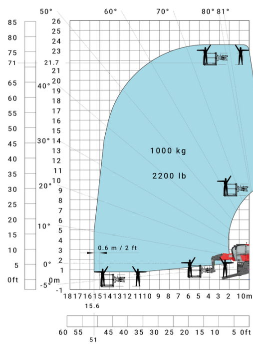
Drehung an abgesenkten Stützen mit 1000 kg Arbeitskorb
