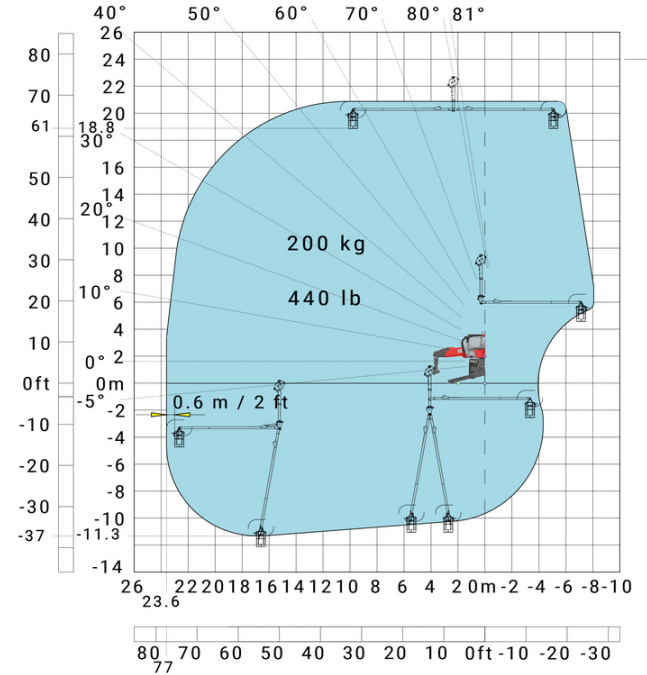
Drehung mit abgesenkten Stützen mit 3D positiv / negativ
