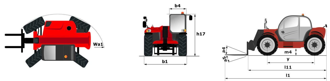
MT 730 H - Rysunek wymiarowy
