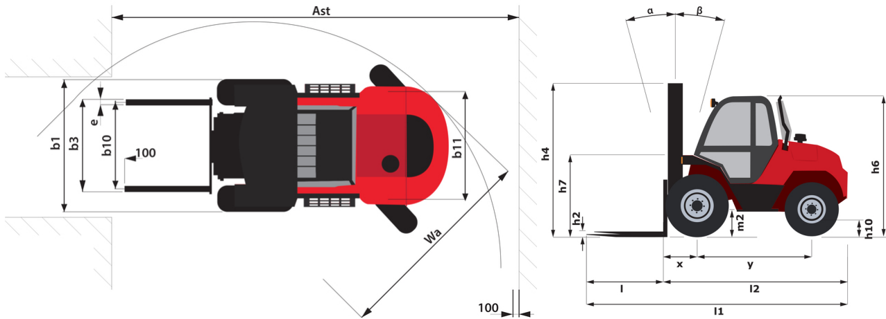
M-X 50-4 - Tekening met afmetingen
