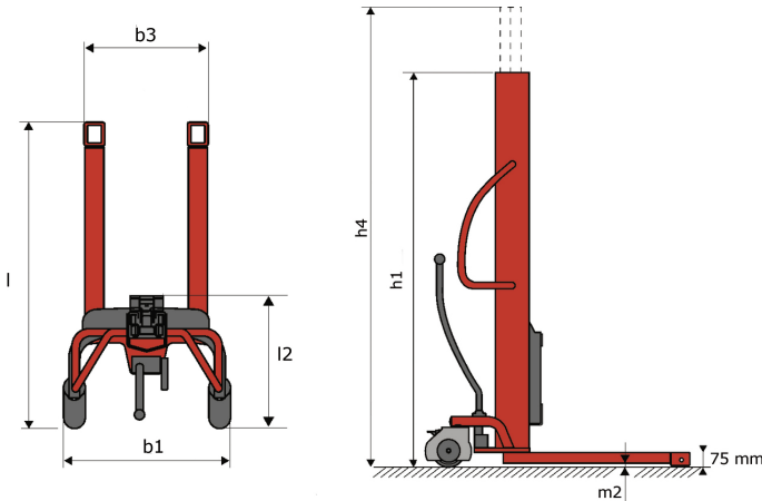
Kleos HM 500 D18 - Tekening met afmetingen
