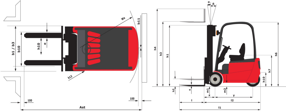
ME 315 - габаритный чертеж
