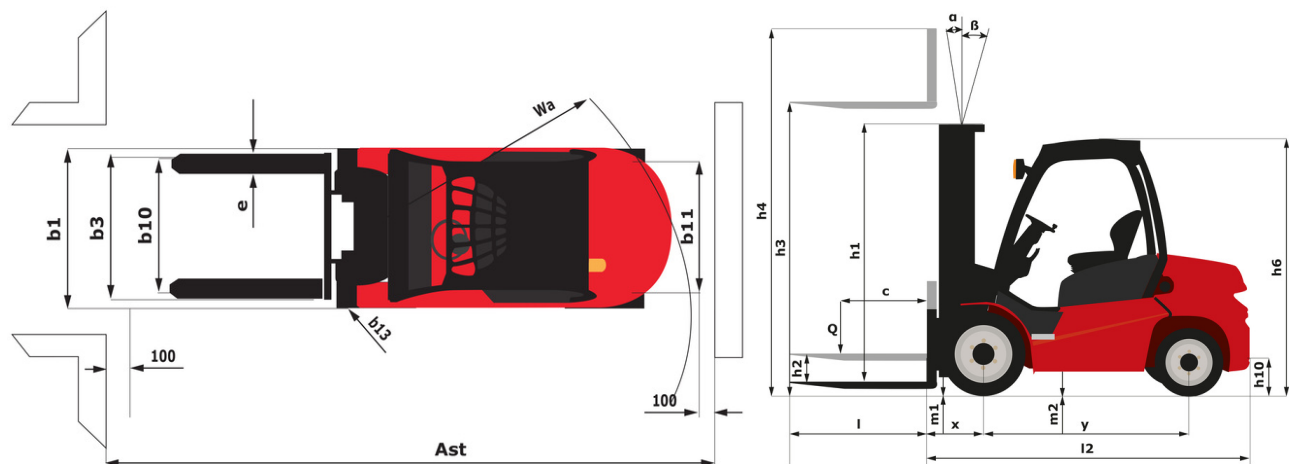
MI 50L G - габаритный чертеж
