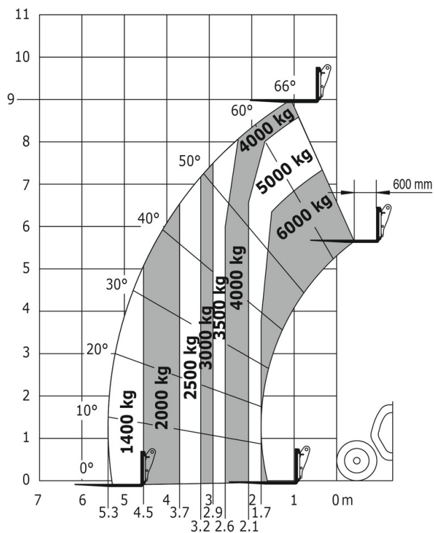
Lastdiagramm „Gelände“ (EN 1459 B)
