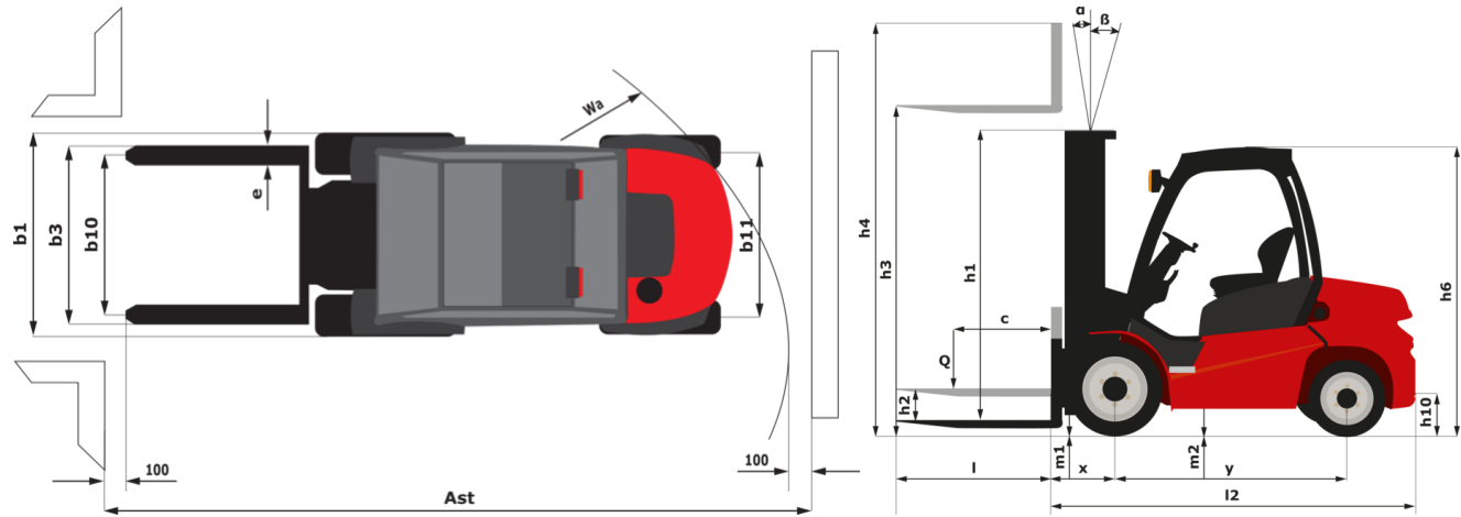
MSI 25 ST5 - Schémas d'encombrement
