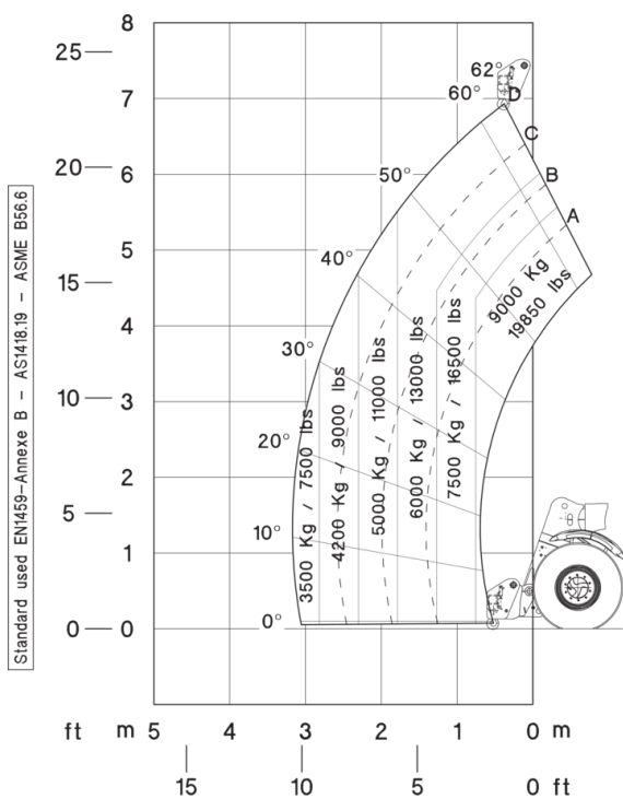
Máquina sobre pneus com jib
