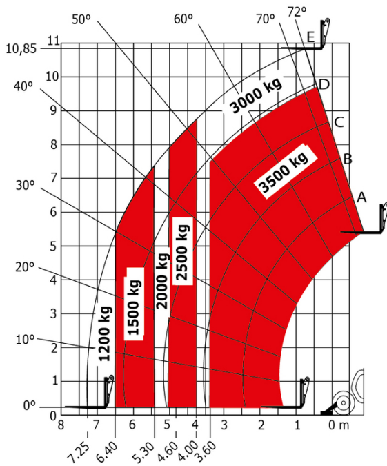
Lastdiagramm
