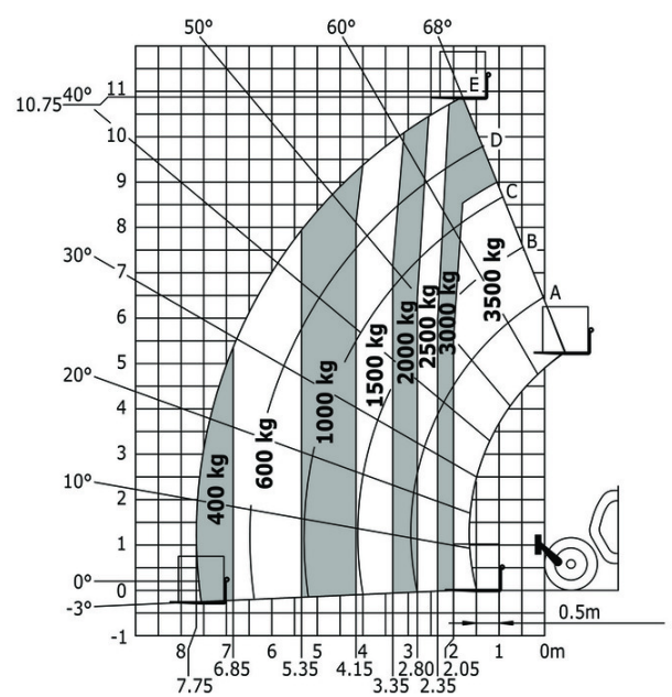
Maszyna na kołach, z widłami - z poziomowaniem
