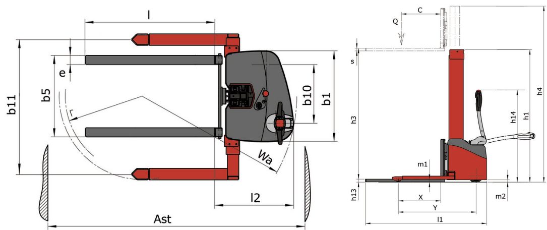
Stacky 10 D28 LE - Tekening met afmetingen
